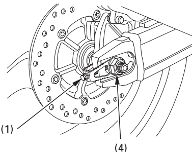
(4) Taka-akselin mutteri
