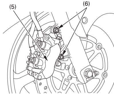
(5) Oikea jarrusylinteri (6) Kiinnityspultit
