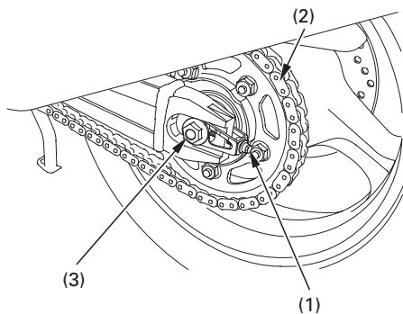
(1) Säätöpultti (2) Toisioketju
