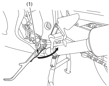
(1) Sivuseisontatuken jousi
